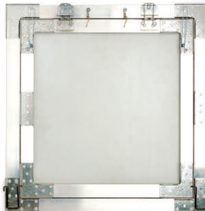
▶ Vista trasera trampilla ALU ▶ Vista de trás alçapão ALU
