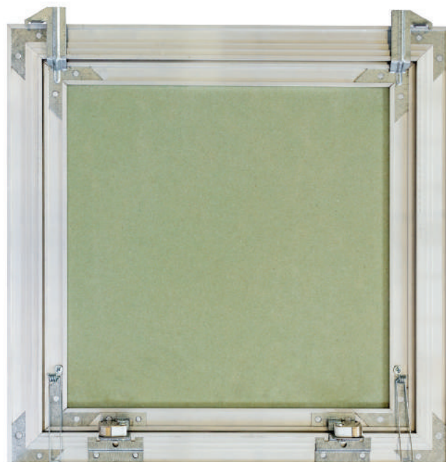
▶ Vista trasera Estanca aire ▶ Vista de trás Estanque ao ar
