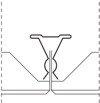
Bandeja Sicilia Clip-In Bisel 3mm
