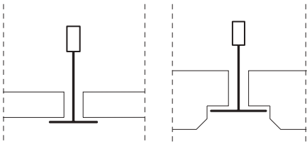
Edge 3 Recto Edge 7 Tegular T24
