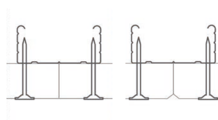
Perfil Oculto Atornillada K0
