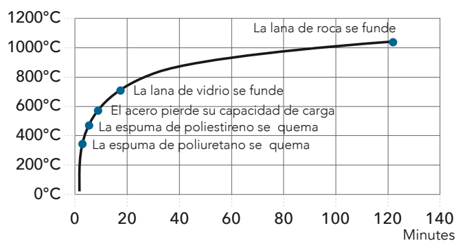
Comportamiento de diferentes materiales conforme a la curva de tiempo/temperatura estándar de la norma ISO 834 sobre resistencia al fuego.
